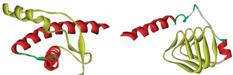
Ett rättveckat prionprotein (till vänster) bredvid ett felveckat. Den gulgröna delen i det felveckade prionproteinet veckas till en så kallad betahelix som kan passa som byggsten i en amyloidfibr.
