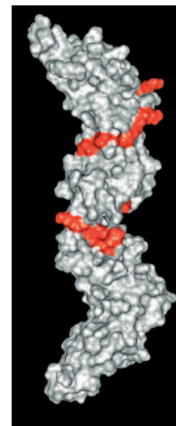
Denna molekylstruktur föreställer en komplementhämmare, KCP, som Annas grupp har identifierat. Den uttrycks av Kaposi's sarcomaassocierat Herpesvirus. De aminosyror som är viktiga för komplementhämmarens funktion visas i rött.
