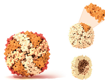
Bilden föreställer proteinet ferritin, som är kroppens lagringsform för järn. Genom att tömma proteinet på järn får man en gjutform som kan användas för att tillverka så kallade "nanomagneterna".
